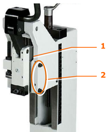
Stelleiste einstellen
